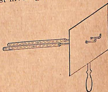
FIG. 18. Double Olfactometer (solid stimuli).
