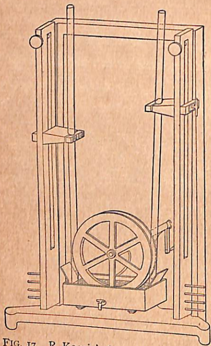
FIG. 17. R. Koenig's Apparatus for the Demonstration of Difference Tones. — Quelques Expériences d'Acoustique , 1882, 165.
